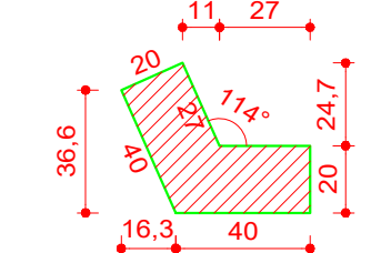
Detalhe 6 (esc. 1:25)
