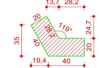
Detalhe 2 (esc. 1:25)
