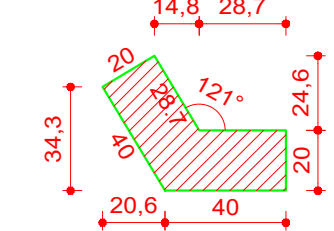
Detalhe 3 (esc. 1:25)
