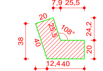
Detalhe 5 (esc. 1:25)
