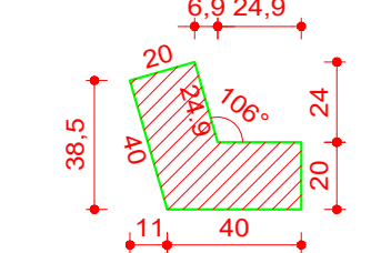
Detalhe 4 (esc. 1:25)
